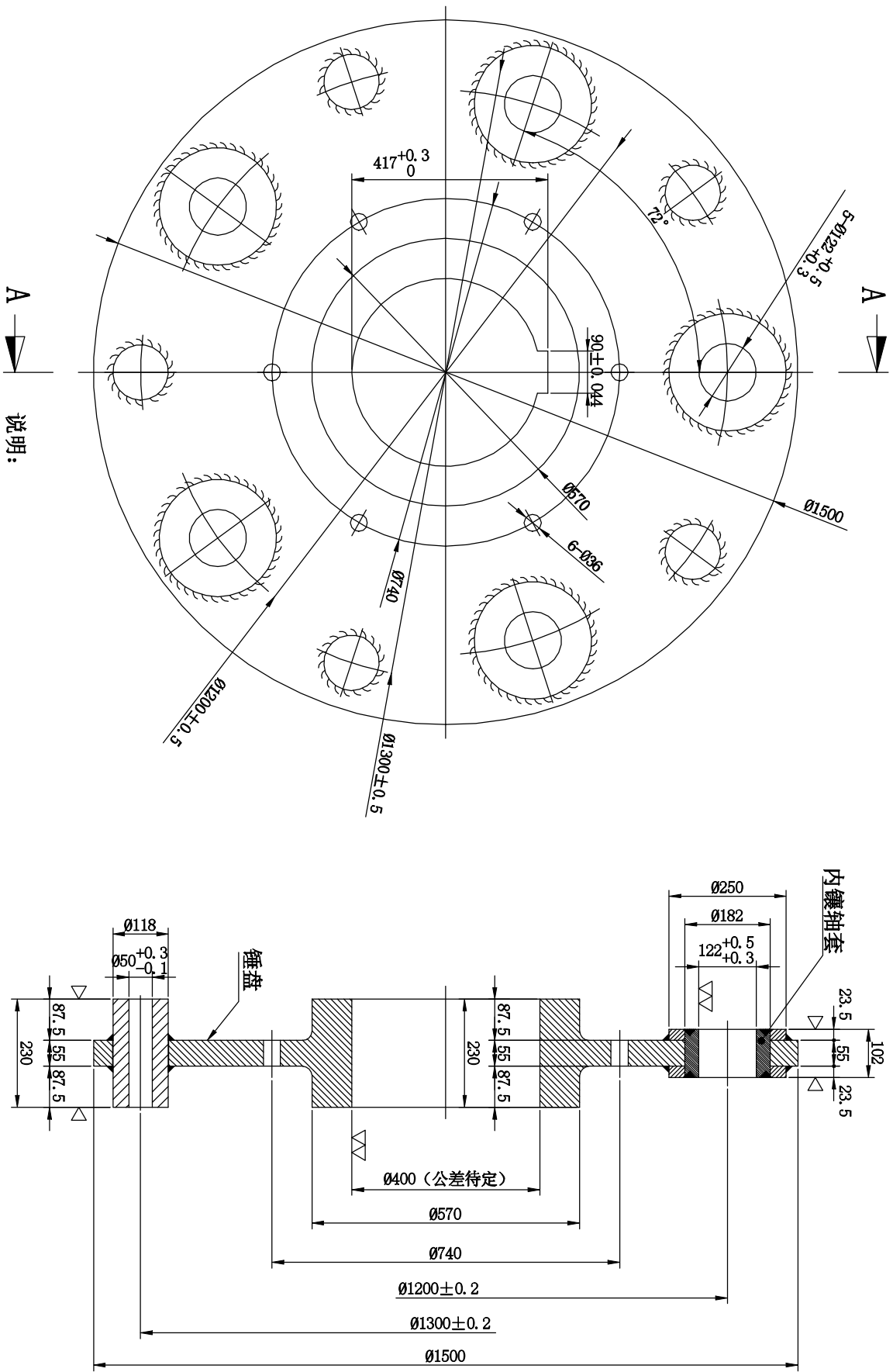
SECTION A-A
